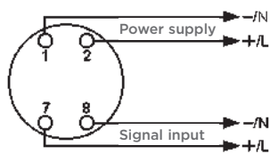
Fig. G Models 007-DA2, 007-DAA LCD digital/analog meter
